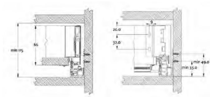
dimensões da cabine p/gaveta
