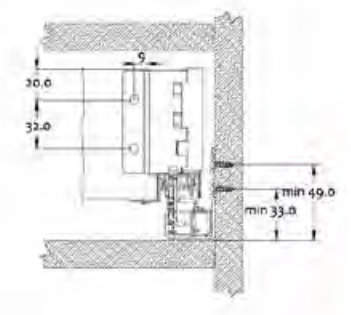
dimensões de instalação do painel traseiro
