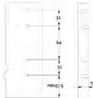
dimensões de perfuração do painel frontal
