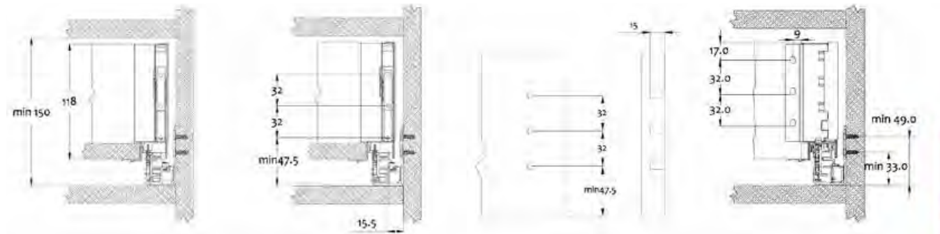
espaço necessário no armário
