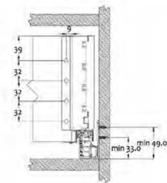
Dimensões de instalação do painel traseiro
