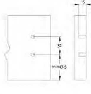
dimensões de perfuração do painel frontal
