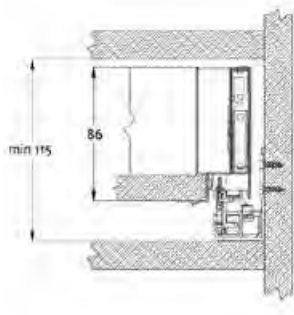
espaço necessário no armário
