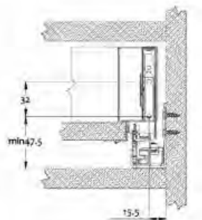
dimensões de instalação do painel do conector frontal
