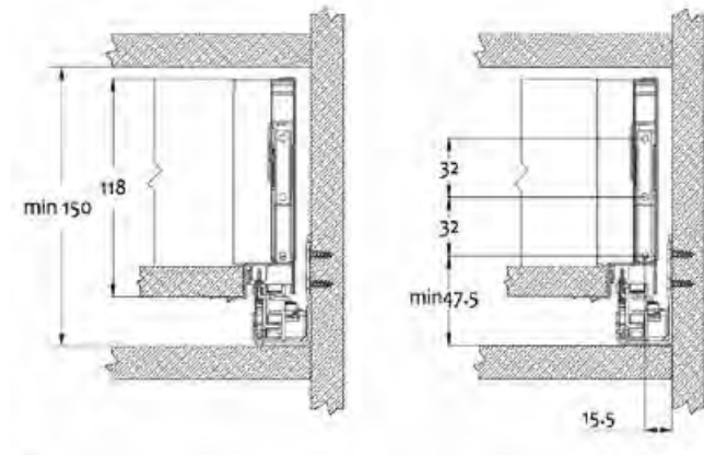
espaço necessário no armário
