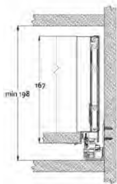
espaço necessário no armário
