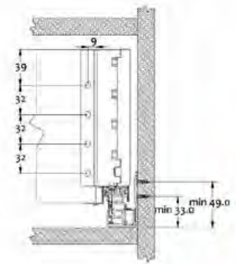
dimensões de instalação do painel traseiro
