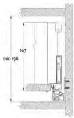
espaço necessário no armário
