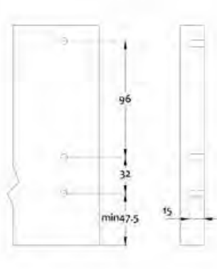
dimensões de perfuração do painel frontal
