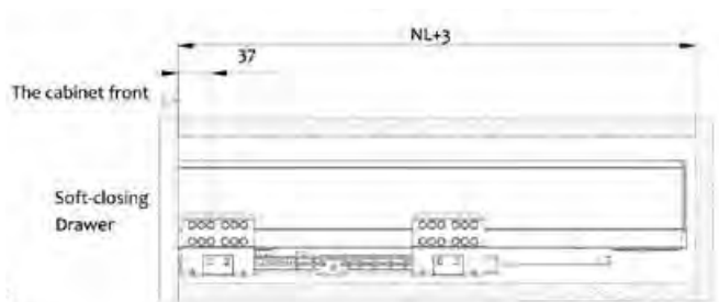
dimensões da cabine p/gaveta
